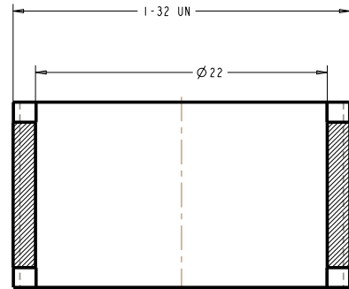
剖面 A-A
